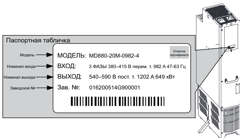
Рис. 2-2 Паспортная табличка
