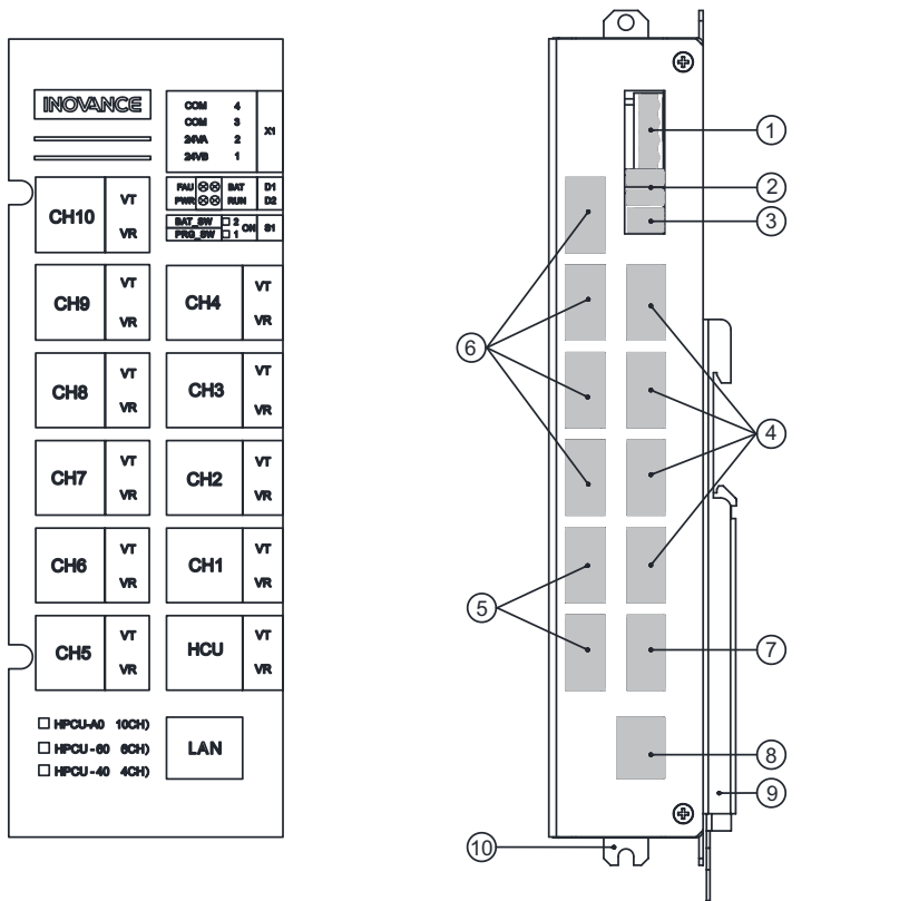
Рис. 5-4 Модуль управления HPCU
