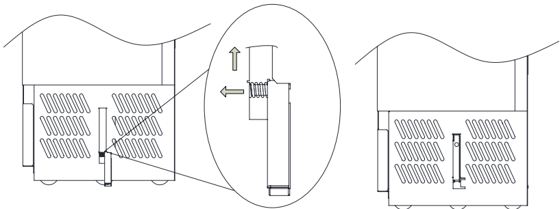
Рис. 6-5 Складывание кронштейна для предотвращения опрокидывания
