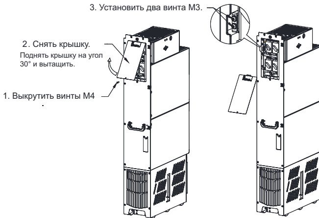
Рис. 4-11 Установка двух винтов М3 на плату VDR
