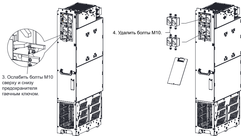
Рис. 6-7 Снятие предохранителя
